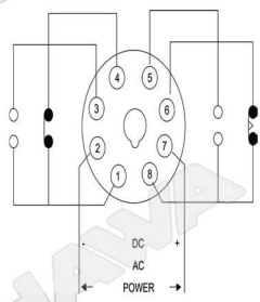
ไทม์เมอร์ 1 ช่วง AH3-2 (คอนแทกหน้า 2 ชุด)
