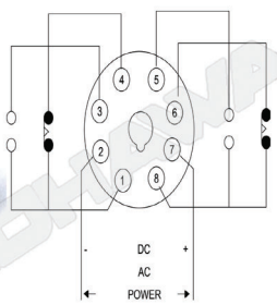
ไทม์เมอร์ 4 ช่วง AH3-(A-E)
