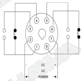
ไทม์เมอร์ 1 ช่วง AH3-2
